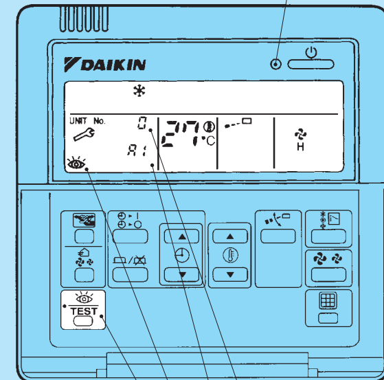
Bouton Inspection/Test Affichage du mode Inspection N° d'unité intérieure présentant un dysfonctionnement Code de dysfonctionnement
